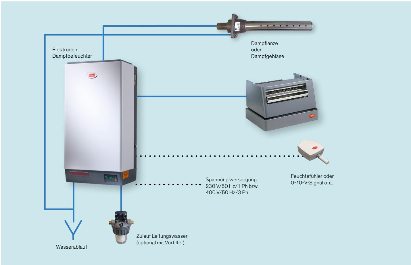
Stulz SupraSteam Anschluss-Systemskizze
